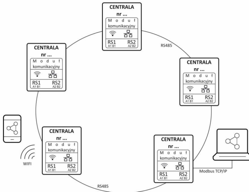
Topologia pierścieniowa RS485 - maks. 16 central, 200 m między urządzeniami
