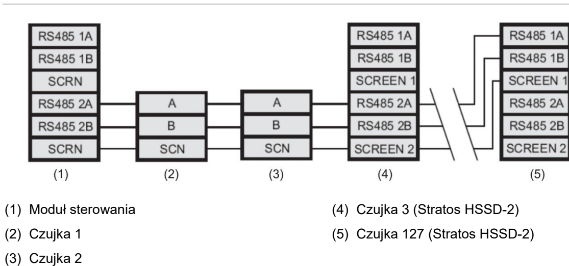
Rysunek 15: Podłączanie czujki do sieci SenseNET
