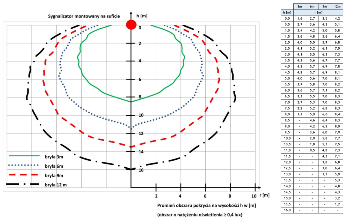
Rys. 7.3.2.1. Obszar pokrycia sygnalizatora SAO-P8/CC, SAO-P8/BC w zależności od wybranej bryły oraz wysokości montażu
