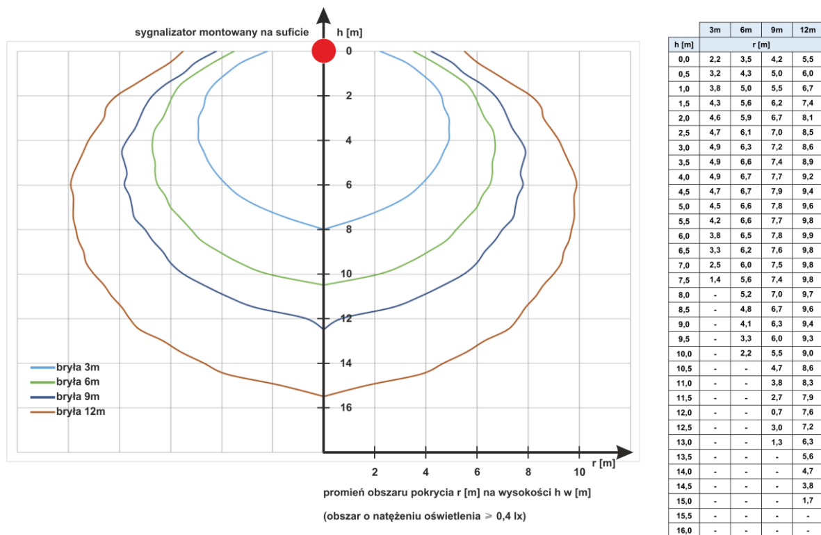
Rys. 7.3.3.1. Obszar pokrycia sygnalizatora SAO-P8/CB, SAO-P8/BB w zależności od wybranej bryły oraz wysokości montażu
