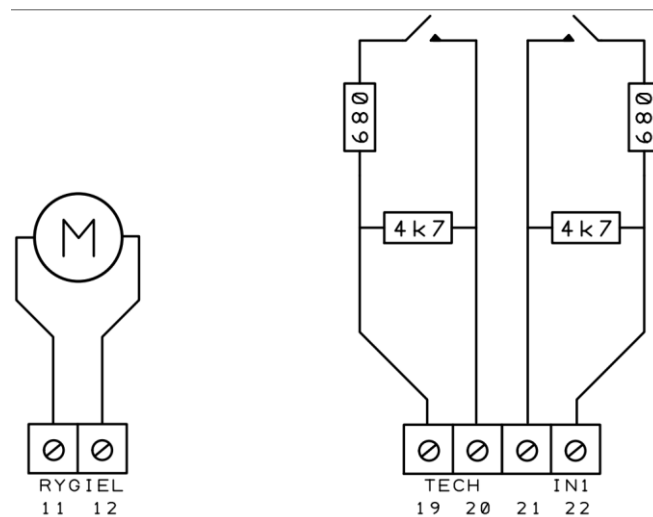
Rysunek 12. Podłączenie siłownika i krańcówek, wersja V2
