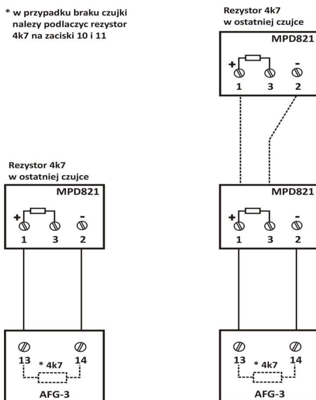
Rysunek 8. Podłączenie czujki dymu: MPD821 (CPD321), MMT860
