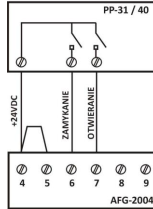
Rysunek 15. Podłączenie przycisku przewietrzania: PPP-31, PP-40
