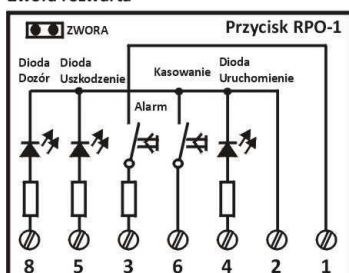
Rysunek 20. Podłączenie przycisku oddymiania: RPO-01
